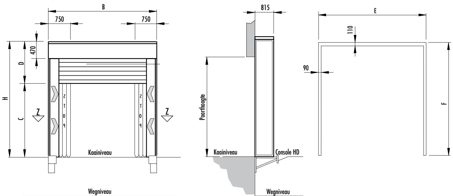
Tekening van model WI
